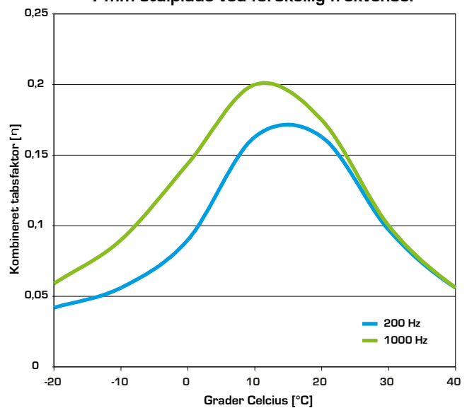
Tabsfaktor for LD13 monteret på en 1 mm stålplade ved forskellig frekvenser
