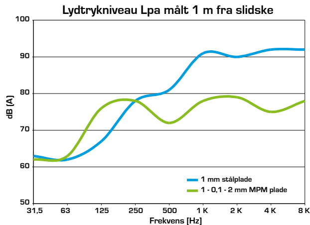
Figur 2. 1/3 oktav analyse af støjen målt ved en transportslidske lavet af henholdsvis 1 mm stålplade og af en MPM plade.
